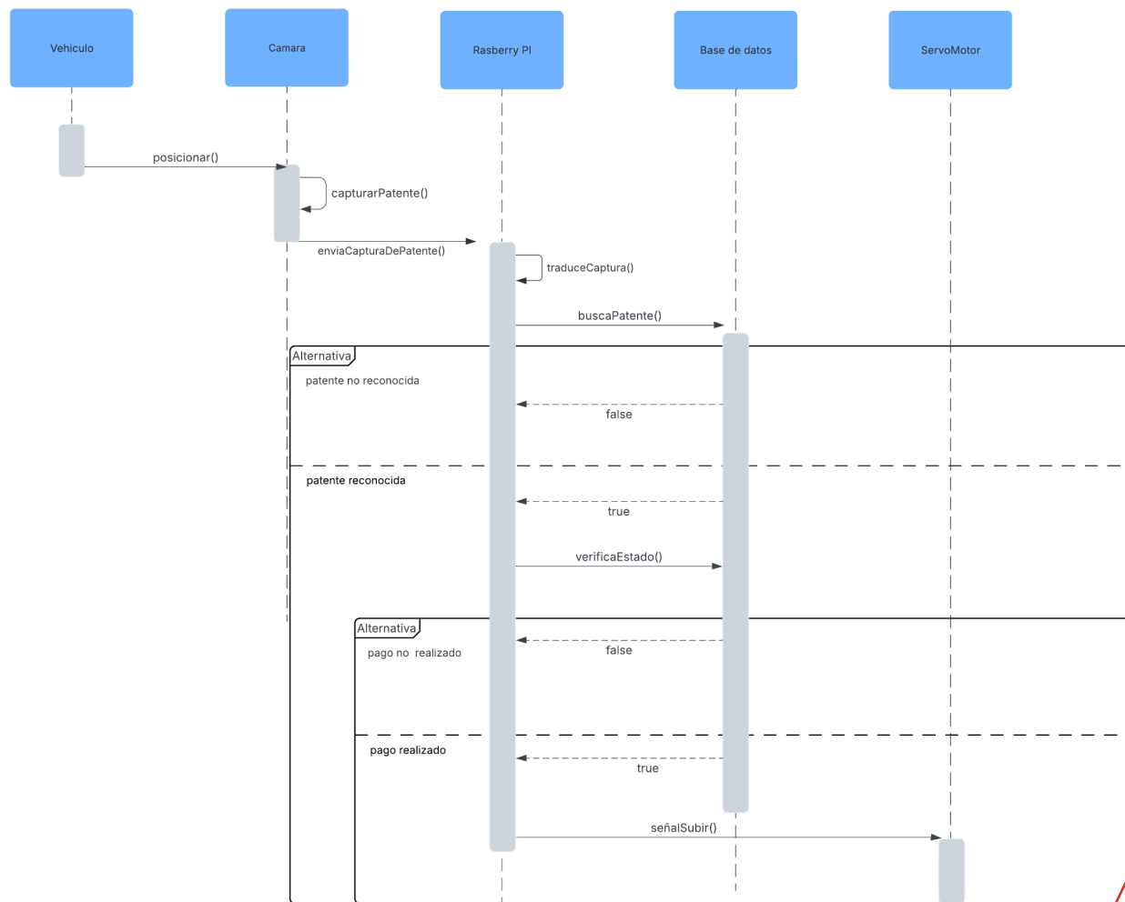
Ilustración 5: Diagrama de secuencia: Gestionar salida vehicular
