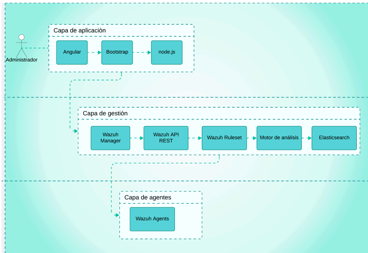
Figura 8: Arquitectura del sistema.
