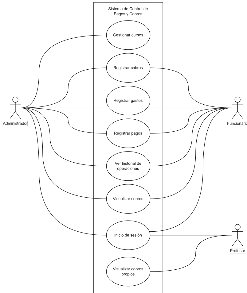
Figura 3: Modelo de casos de uso
