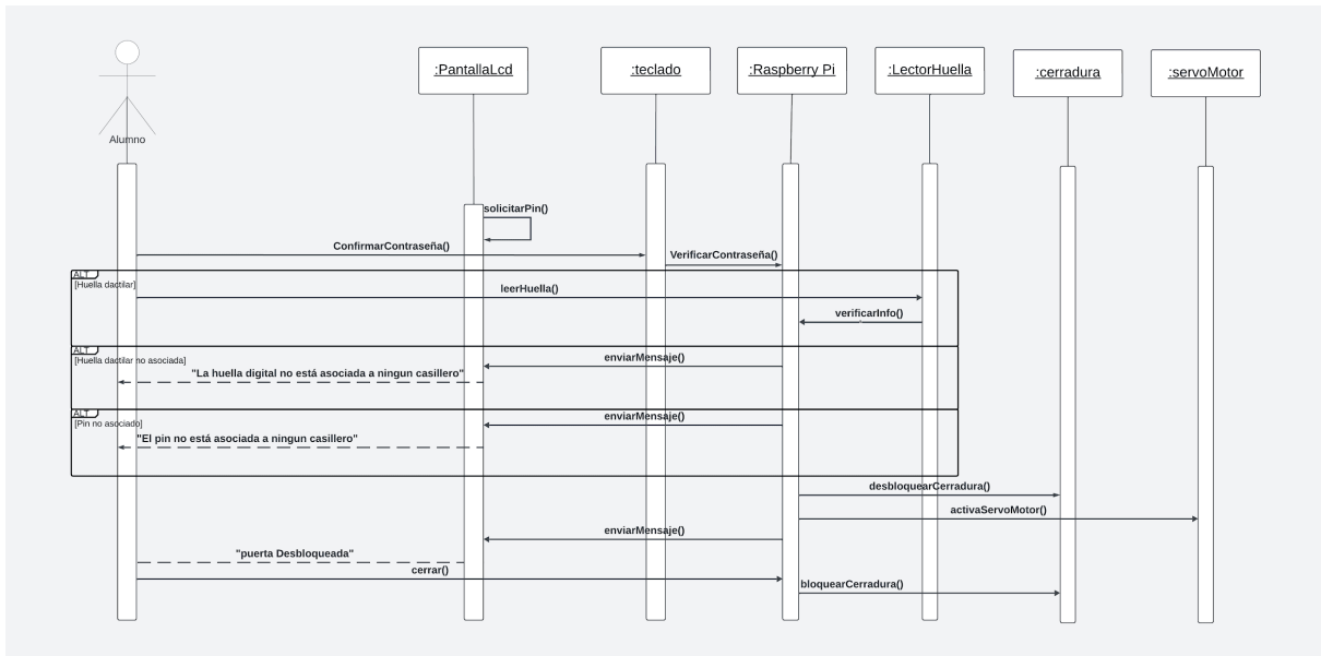
Ilustración 8 Diagrama de Secuencia: Abrir Casillero
