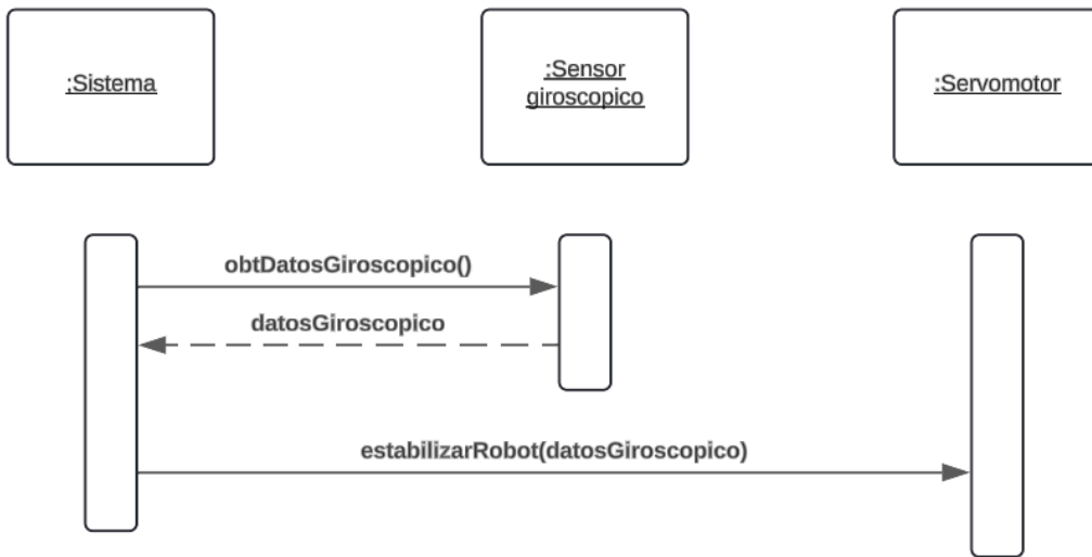
fig n°6: Diagrama de secuencia que modela el CUS estabilizar robot.
