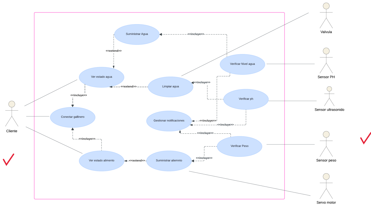
Ilustración 9 : Diagrama Caso de Uso de Contexto
