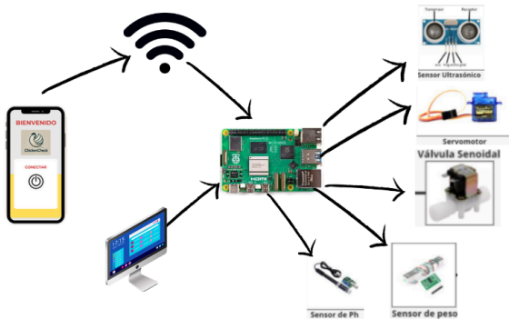
Ilustración 3: Descripción Arquitectura 2
