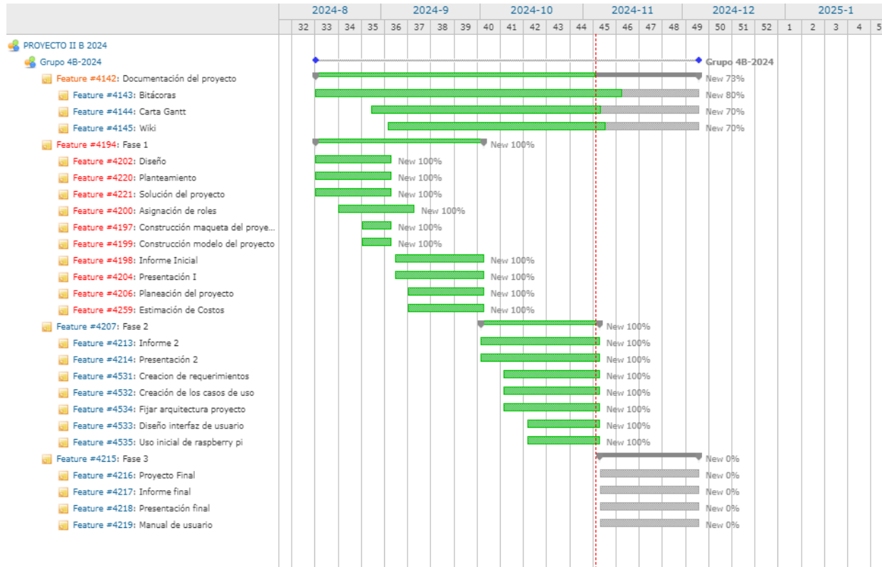
Ilustración 1: Carta Gantt.
