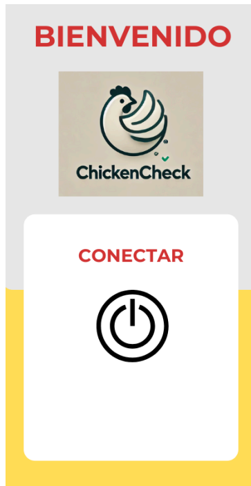
Ilustración 4: Inicio
