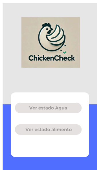
Ilustración 5: Menú
