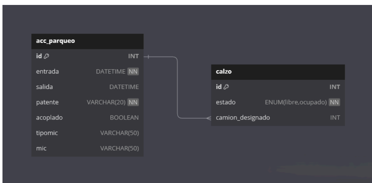
Figura 8: Modelo entidad-relación.
