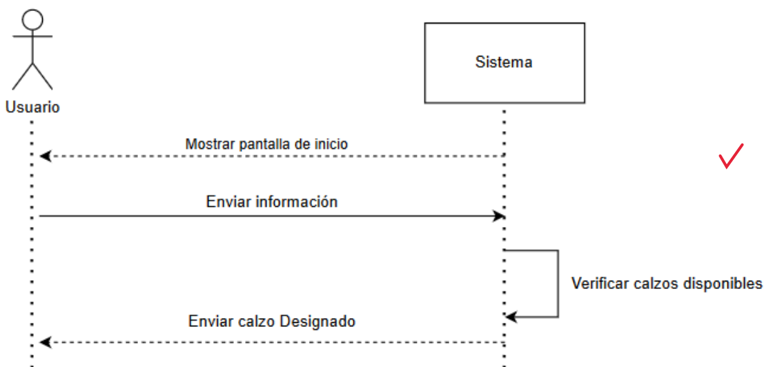
Figura 4: Diagrama de Secuencia Asignación calzo.
