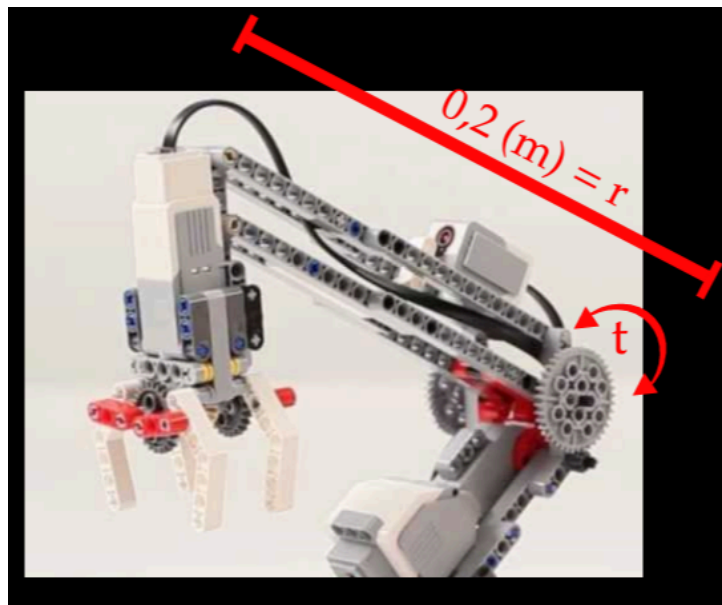
Diagrama 6: Análisis físico de la garra y el torque que produce sobre el objeto que toma
