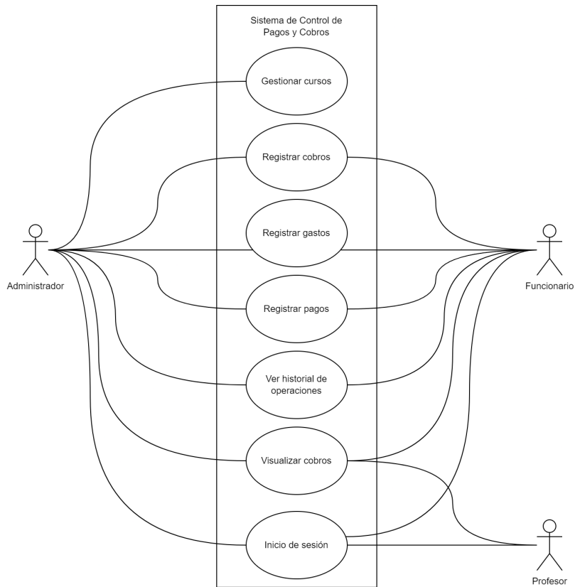
Figura 3: Modelo de casos de uso
