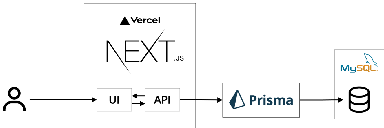
Figura 7: Arquitectura del sistema
