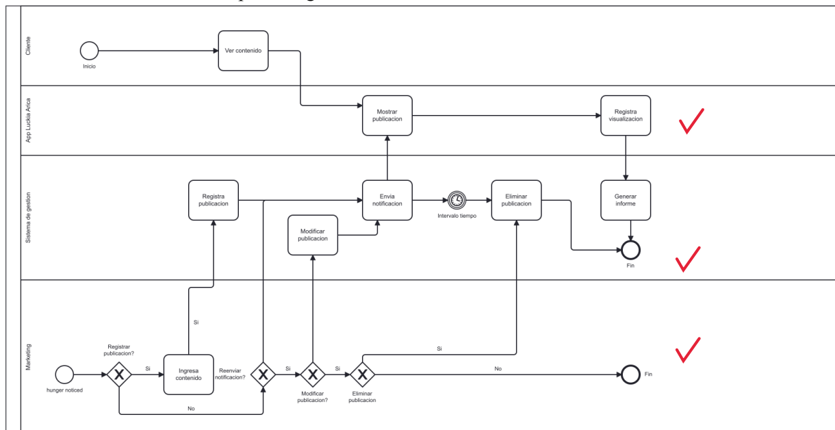
Ilustración 3: Modelo de proceso del funcionamiento del sistema App Luckia Arica.
