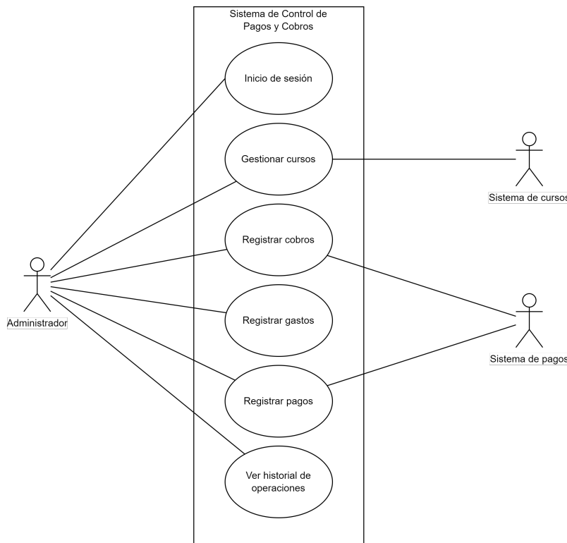
Figura 3: Modelo de casos de uso
