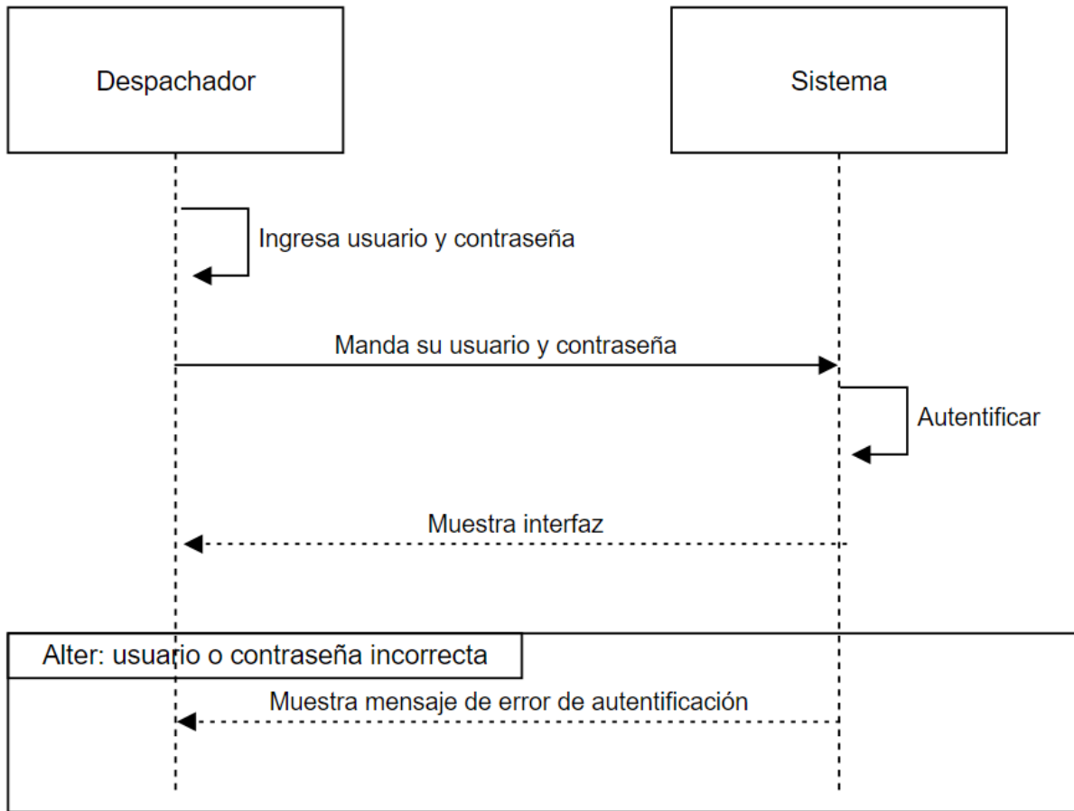
Figura 4: Diagrama Iniciar Sesión.
