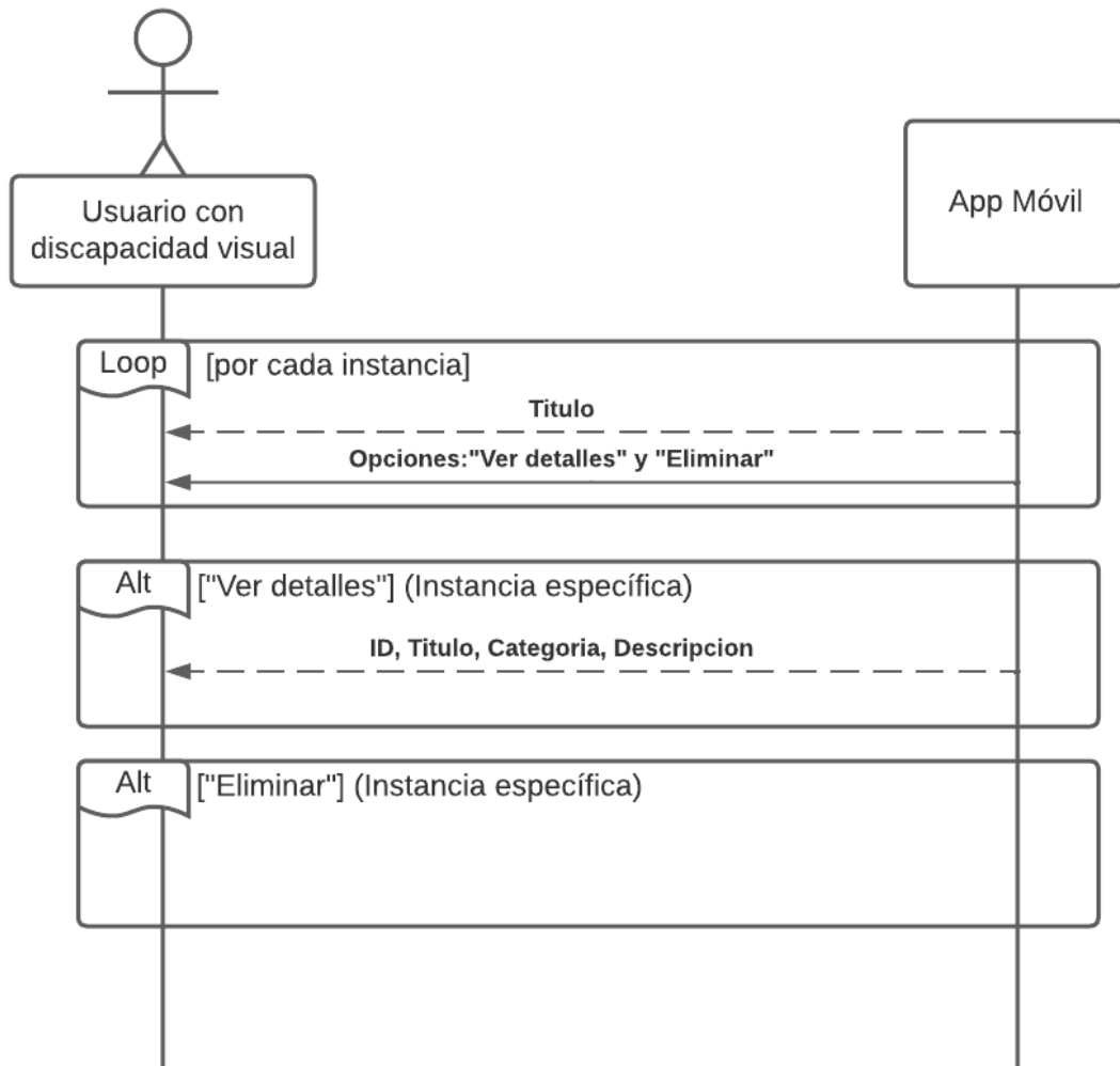
Ilustración 10: Listar Registros NFC (App Móvil) - Diagrama nivel 0.
