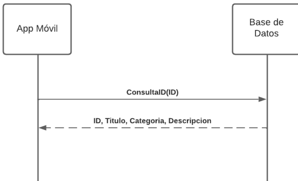
Ilustración 16: Retornar instancia de la Base de Datos - Diagrama nivel 0.
