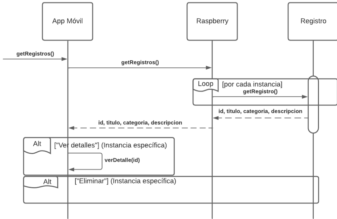
Ilustración 11: Listar registros NFC (App Móvil) - Diagrama nivel 1.
