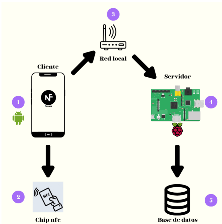
Ilustración 4: Descripción de la Arquitectura.
