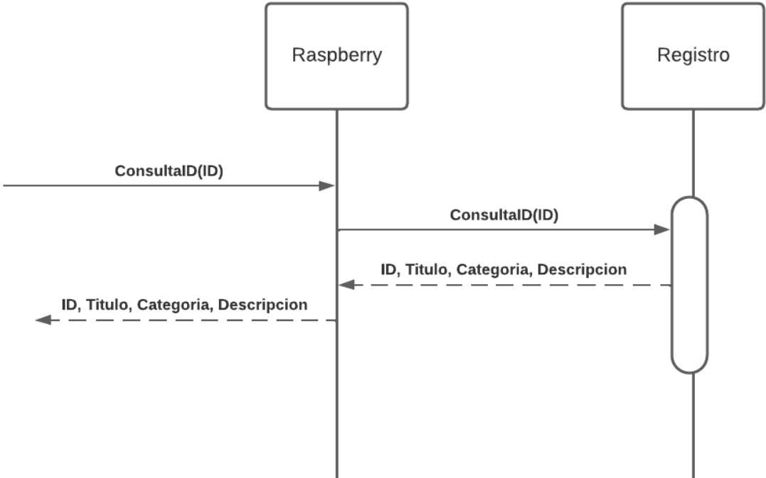
Ilustración 17: Retornar instancia de la Base de Datos - Diagrama nivel 1.
