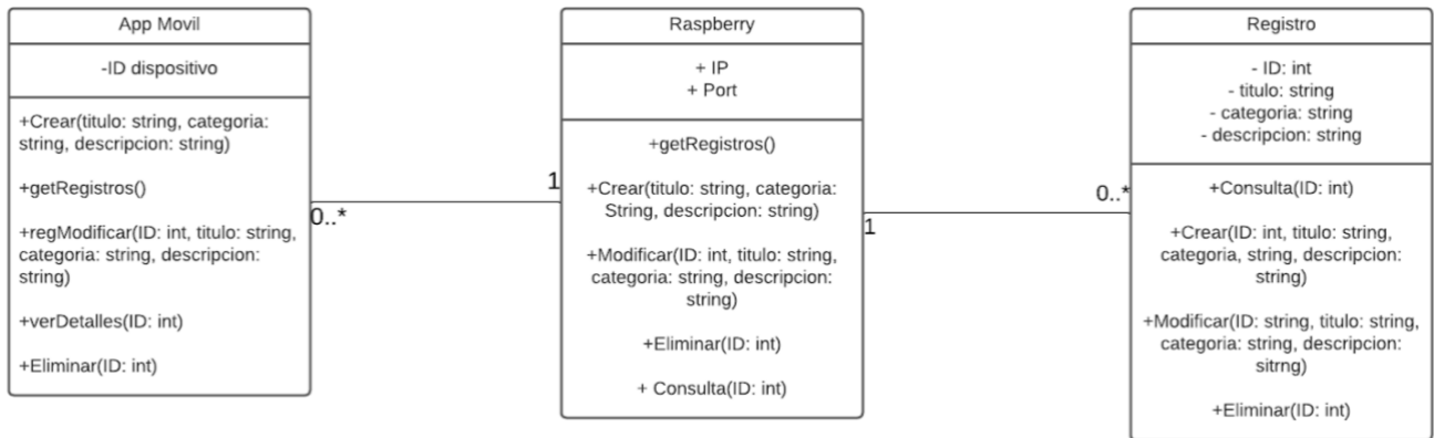
Ilustración 18: Diagrama de clases.
