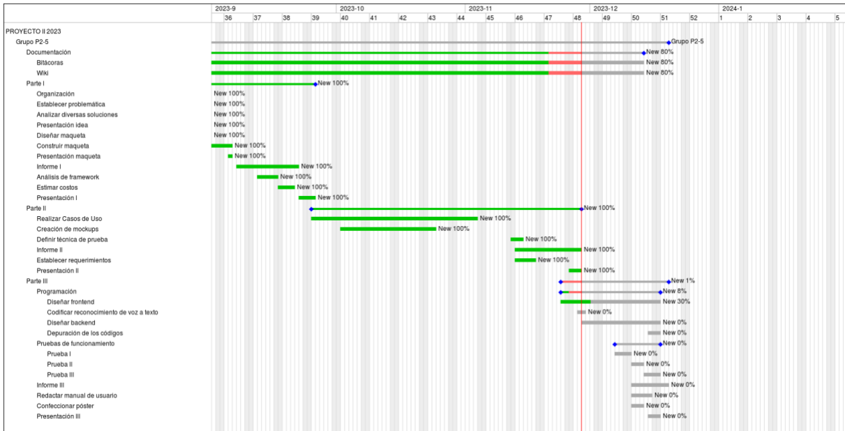
Ilustración 3: Carta Gantt.
