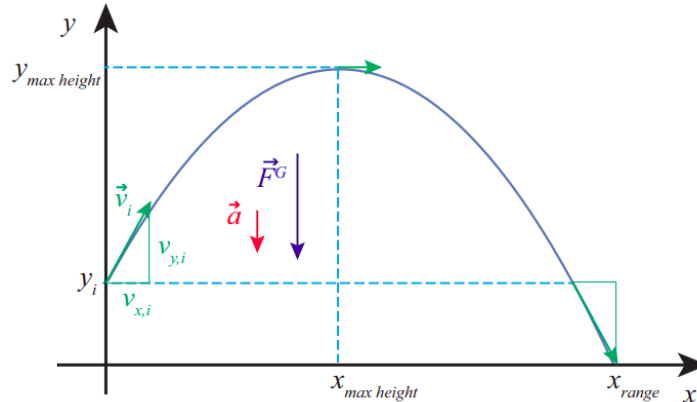
Ilustración 4: Movimiento parabólico.
