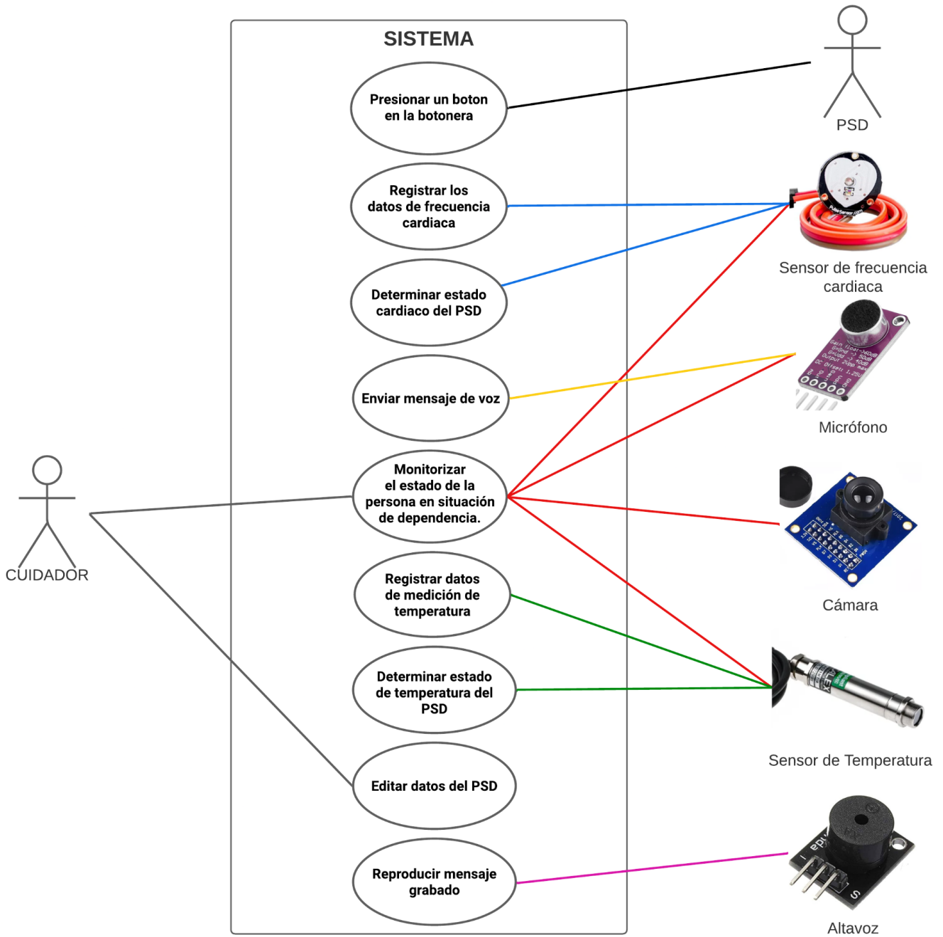
Diagrama de casos de uso base
